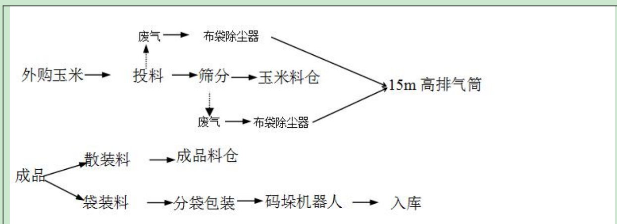
图 2-7 技改项目生产工艺流程图及产污环节
