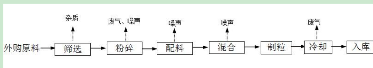
图2-6 技改完成后生产工艺流程图及产污环节
